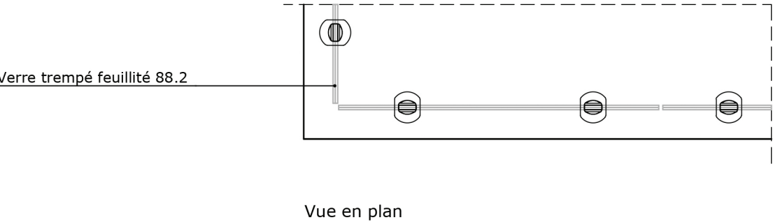
Détail de jonction à l'angle GlassFit CC-782 Sans main-courante Échelle 1:20
