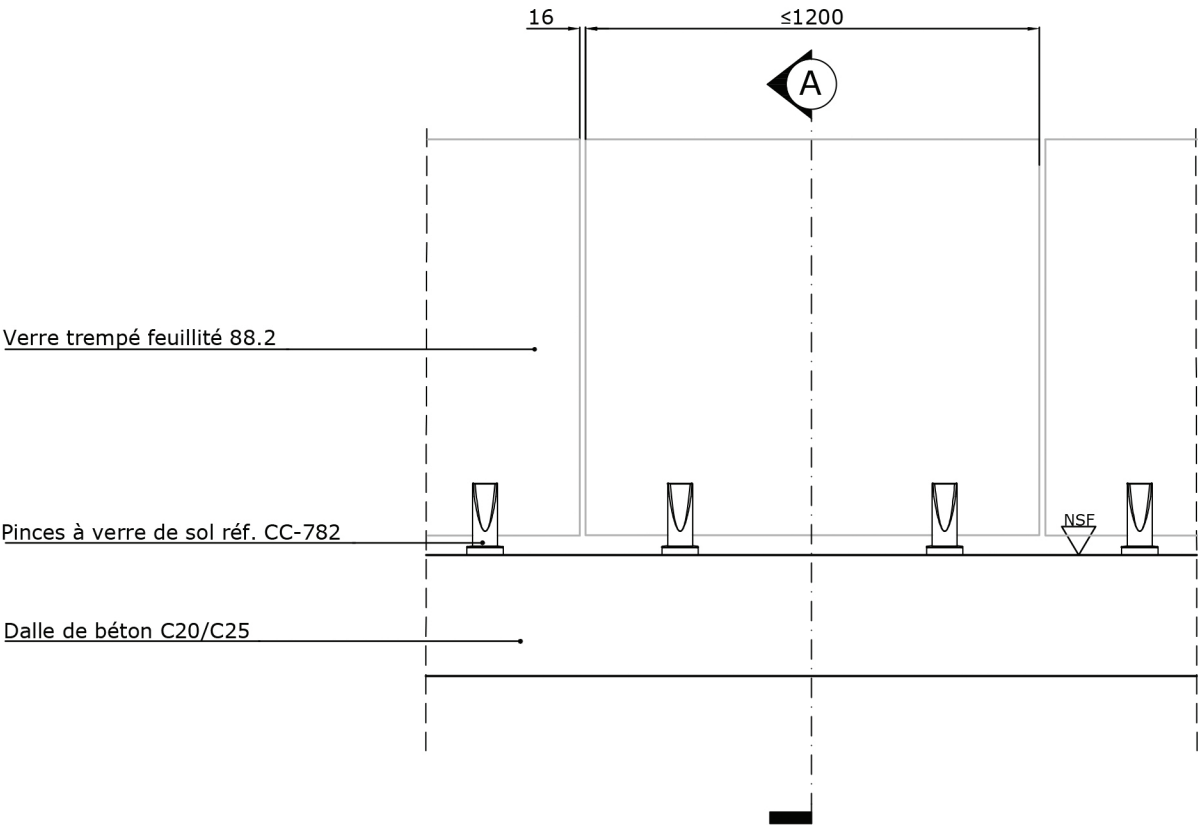
Détail tronçon horizontal type GlassFit CC-782 Sans main-courante Échelle 1:20
