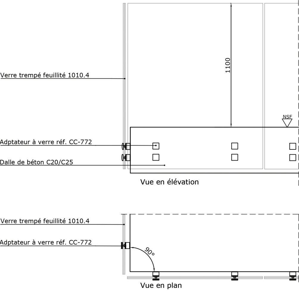
Détail de jonction à l'angle GlassFit CC-772 Sans main-courante Échelle 1:20
