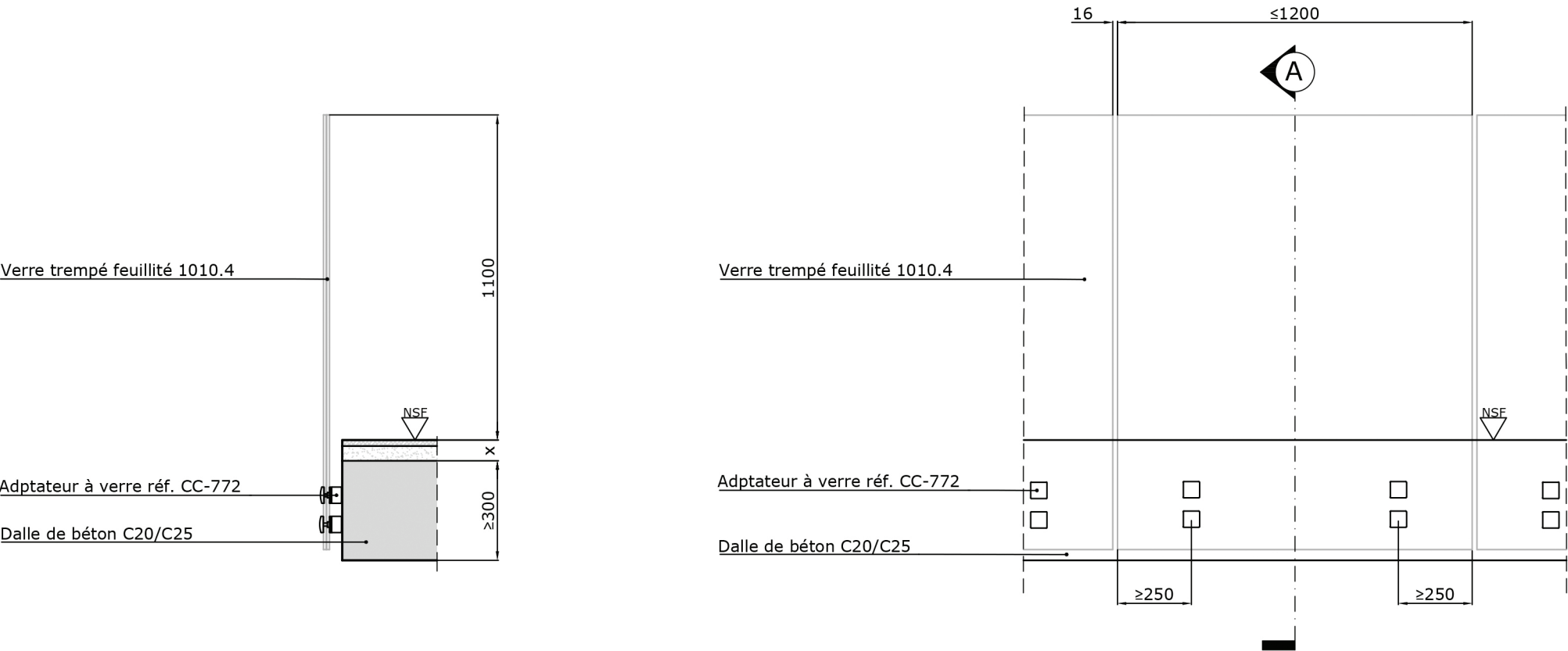
Coupe A-A GlassFit CC-772 Sans main-courante Échelle 1:20
