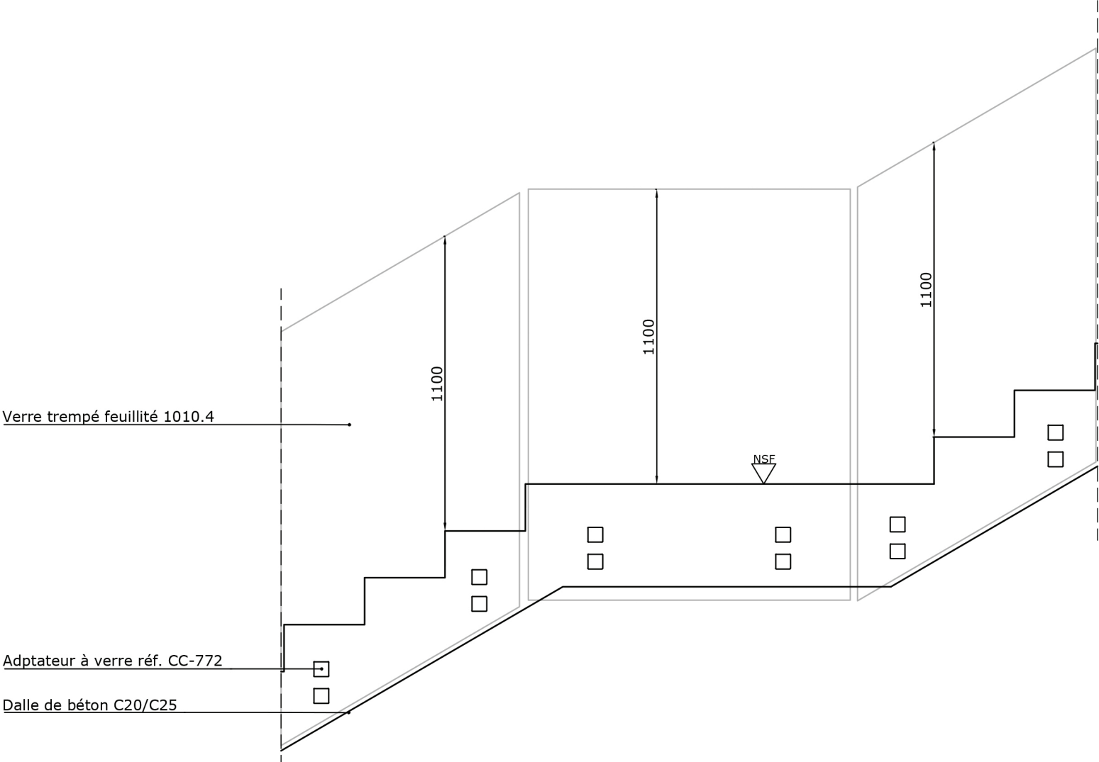
Détail jonction tronçons inclinés avec tronçons horizontals GlassFit CC-772 Sans main-courante Échelle 1:20
